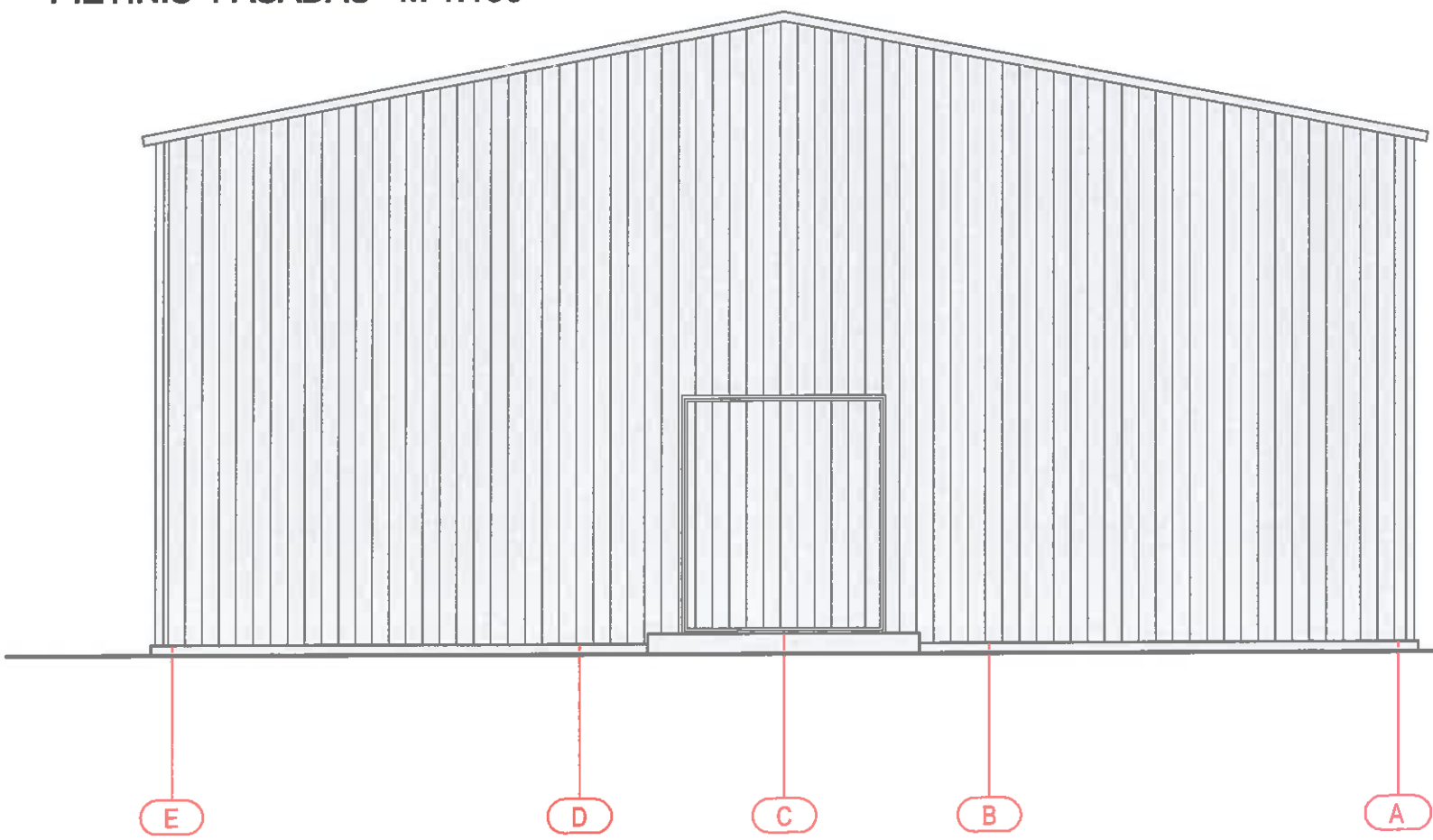
PIETINIS FASADAS M 1:100
