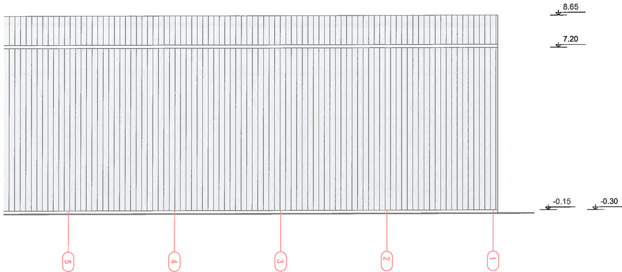
VAKARINIS FASADAS M 1:100
